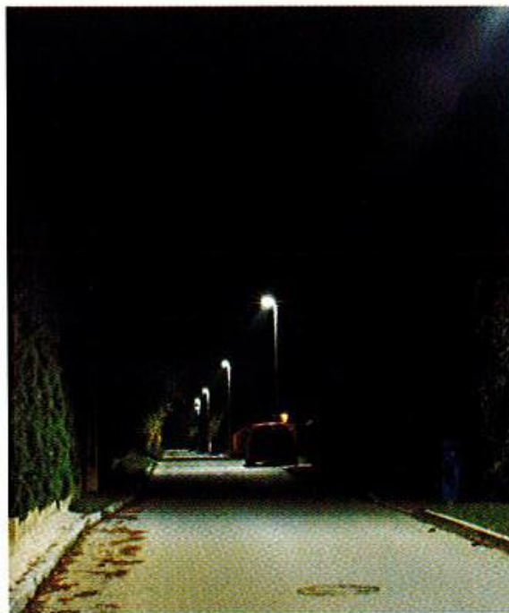
Oświetlenie uliczne solarne w miejscowości Maszewo Duże, ul. Morelowa. Lampy solarne typu MEWA20.
