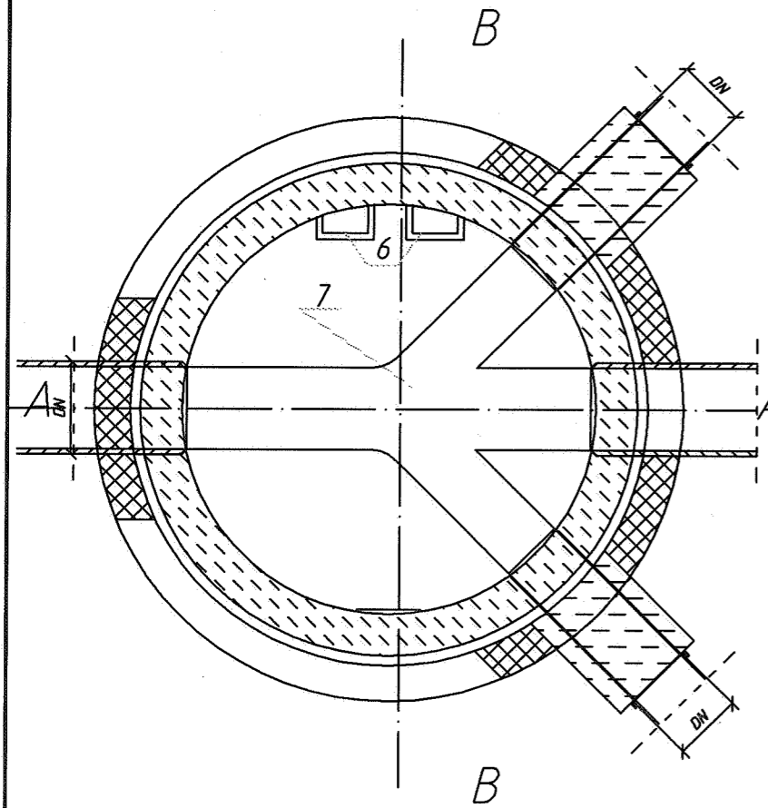
Rzut C-C
