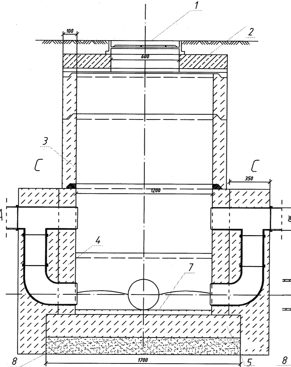
Rzut B-B
