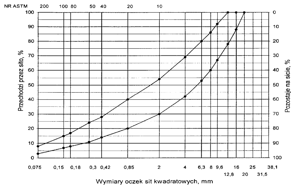
Rys. 2. Krzywe graniczne uziarnienia mieszanki mineralnej BA od 0 do 16 mm do warstwy wiążącej nawierzchni drogi o obciążeniu ruchem KR1
