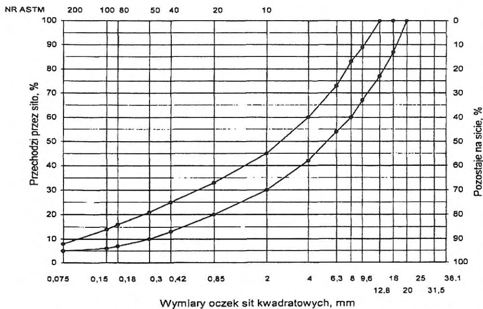
Rys. 1. Krzywe graniczne uziarnienia mieszanki mineralnej BA od 0 do 25 mm do warstwy wiążącej,
