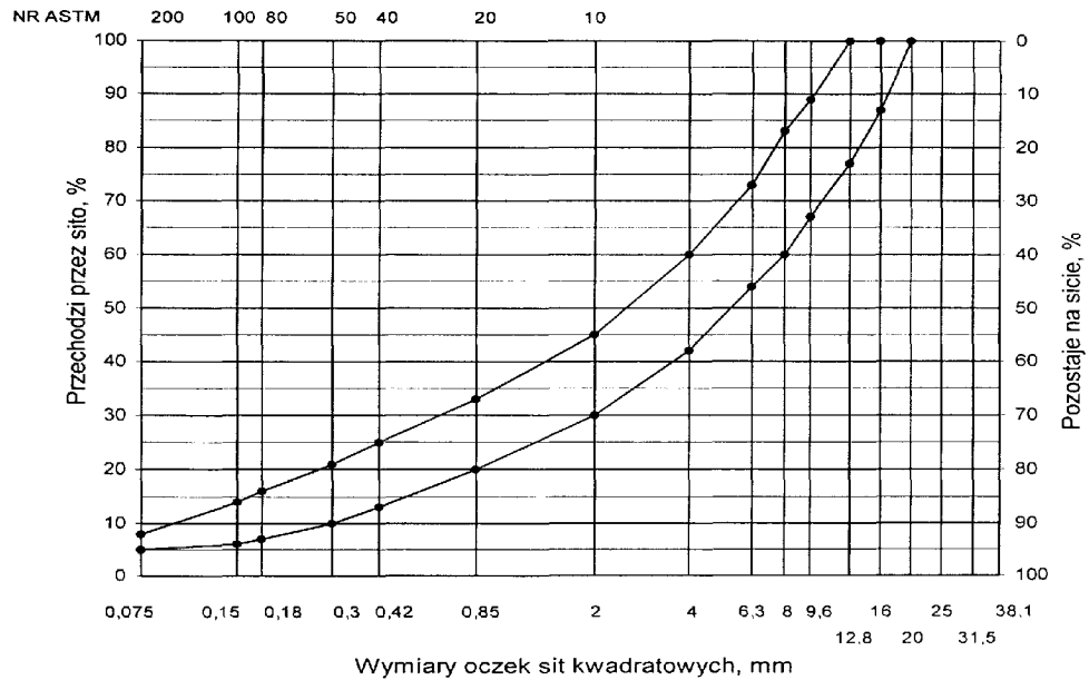
Rys. 1. Krzywe graniczne uziarnienia mieszanki mineralnej BA od 0 do 25 mm do warstwy wiążącej, nawierzchni drogi o obciążeniu ruchem od KR 46. Wymagania wobec warstwy wiążącej z betonu asfaltowego
