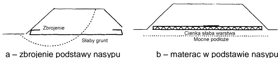
Rys. 2.2. Przykłady zbrojenia nasypów geosyntytykami
