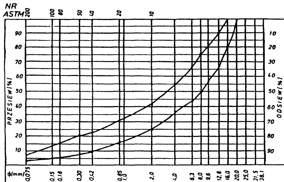
Rys. 12. Krzywe graniczne uziarnienia mieszanki mineralnej 0+20 mm do warstwy
