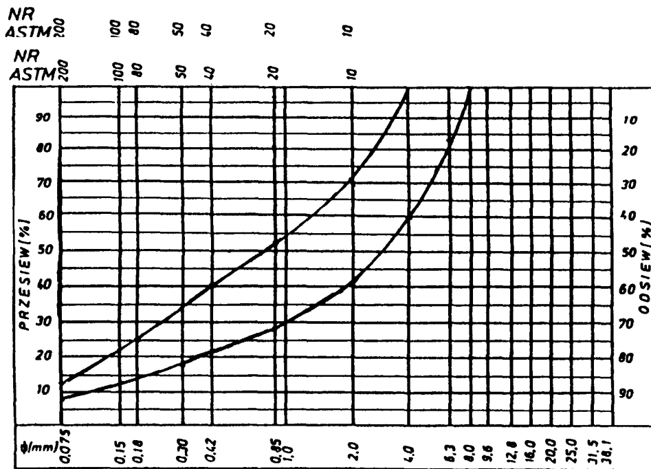
65 Rys. 3. Krzywe graniczne uziarnieni a mieszanki mineralnej 0÷8, 0÷6,3 mm do warstwy ścieralnej z betonu asfaltowego dla KR 1-2
